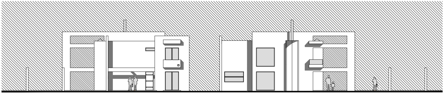
Νότια όψη
