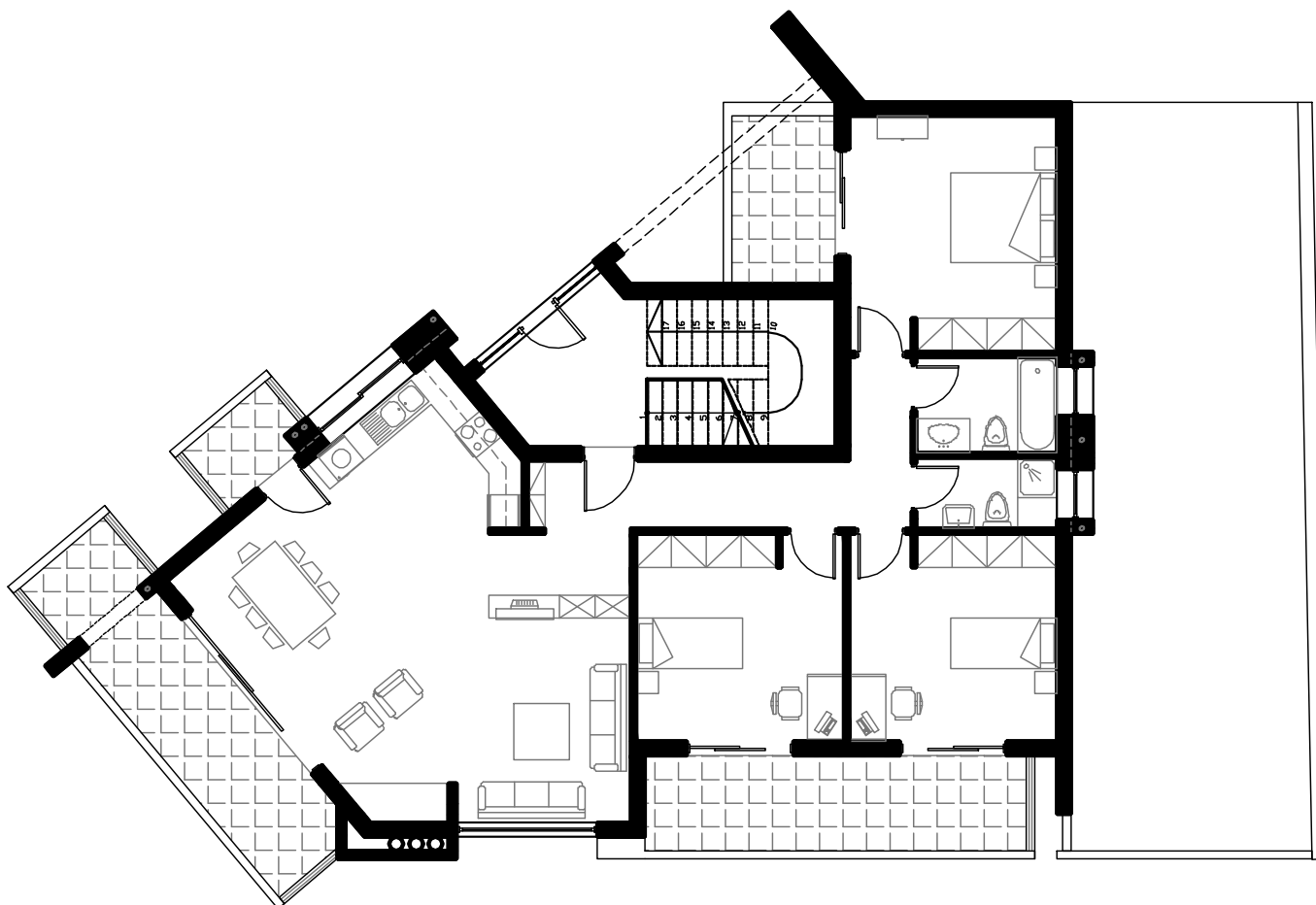
Κάτοψη Ισογείου
