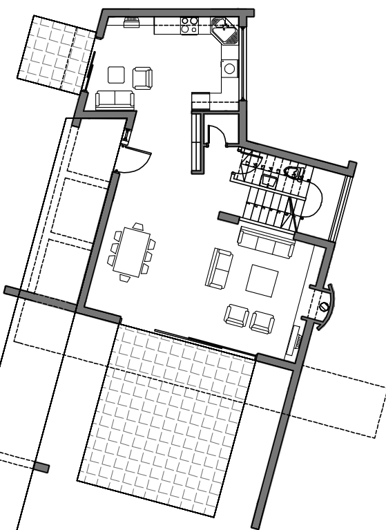
Κάτοψη Ισογείου
