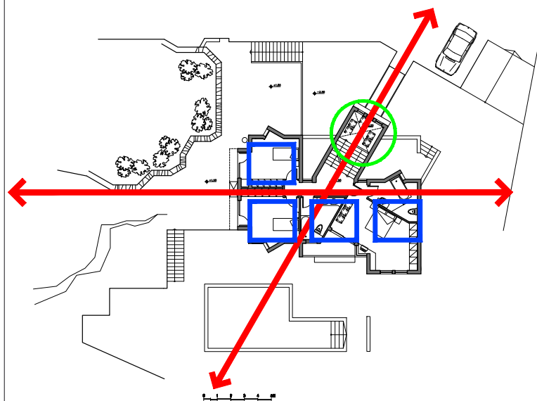
Οργάνωση Ορόφου
