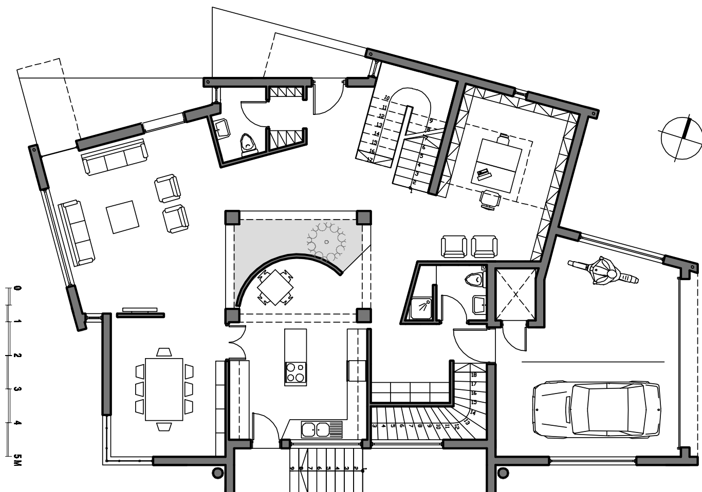
Κάτοψη Ισογείου
