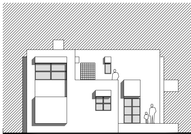
Δυτική όψη
