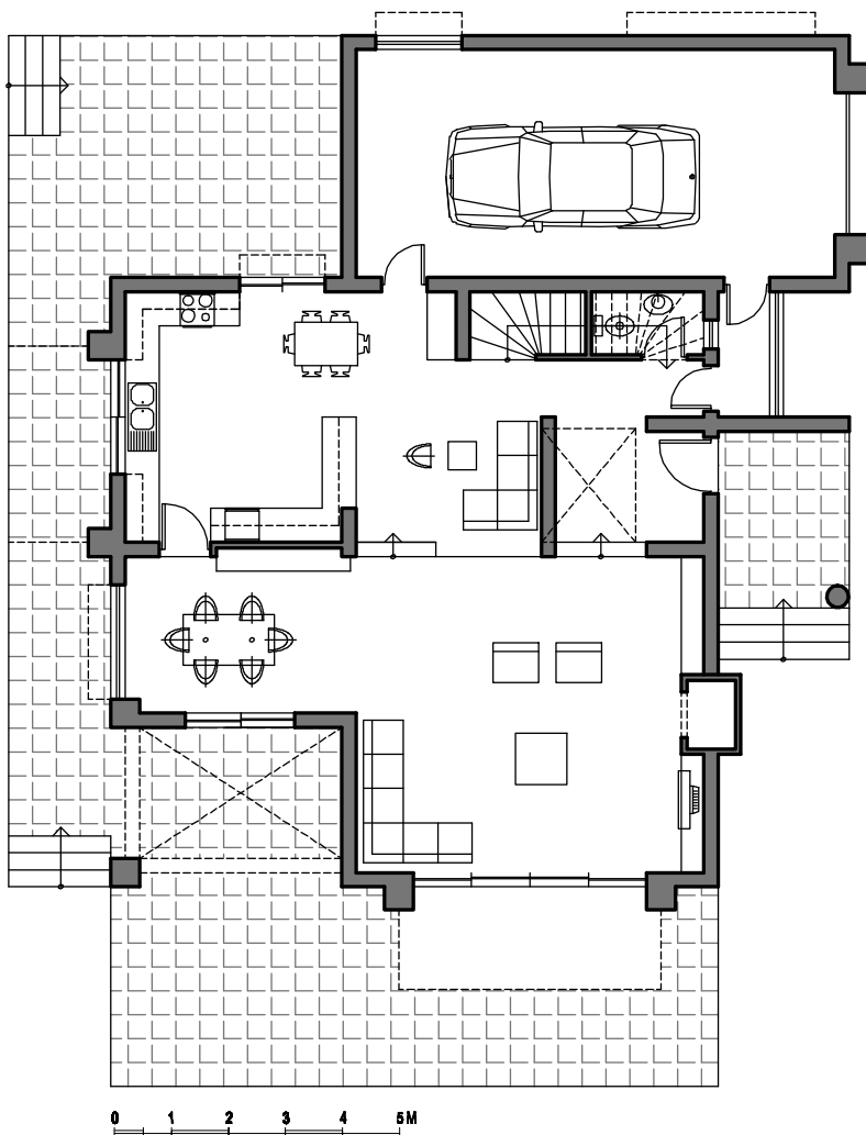
Κάτοψη Ισογείου
