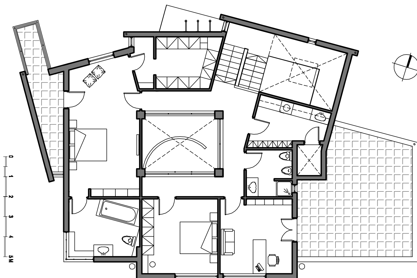
Κάτοψη Ορόφου
